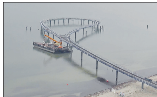
Am Mittwochmorgen, 22. Mai, hat sich der Arbeitsponton unter der Brücke verkeilt. (Foto: Webcam/TSNT GmbH)
