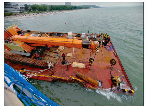
Blick von der Seebücke auf den gestrandeten Arbeitsponton, in dem Taucher versuchen, die beschädigten Kammern zu reparieren. (Foto: René Kleinschmidt)
