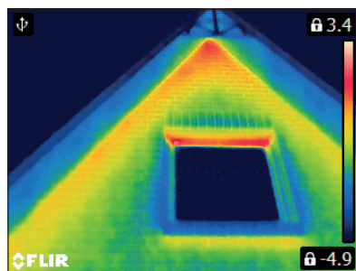
Die Aufnahme macht es deutlich: An den roten Stellen des Gebäudes geht Wärme verloren. Fotos: Gemeinde Stockelsdorf
