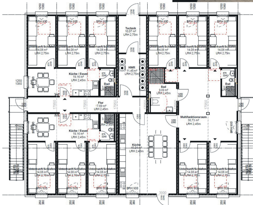
Das ist der Grundriss des Erdgeschosses.
